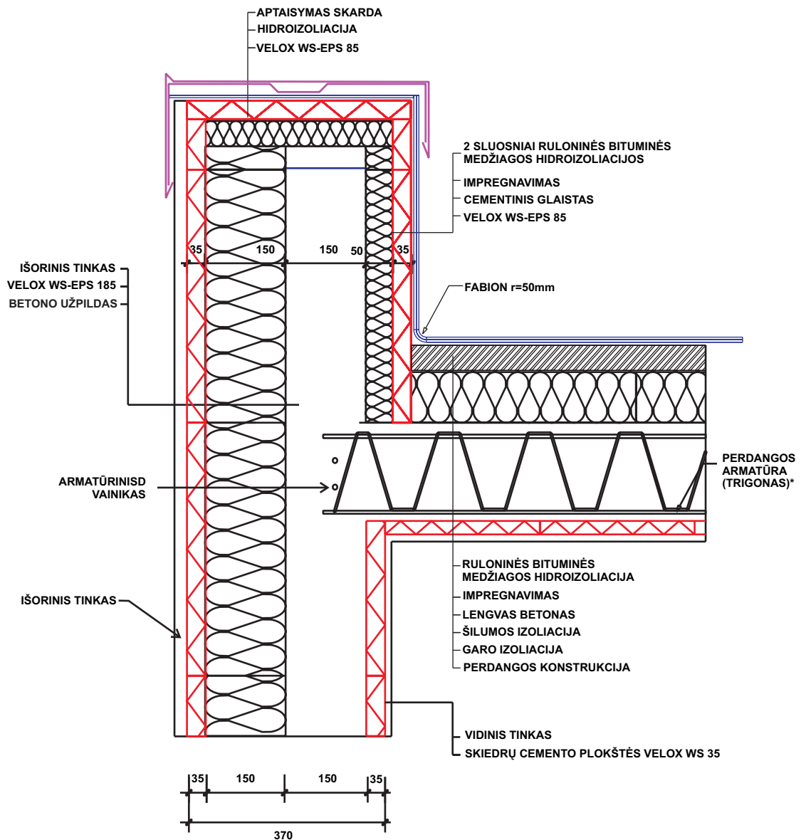
SIENOS STRUKTŪRA VELOX UL 37
