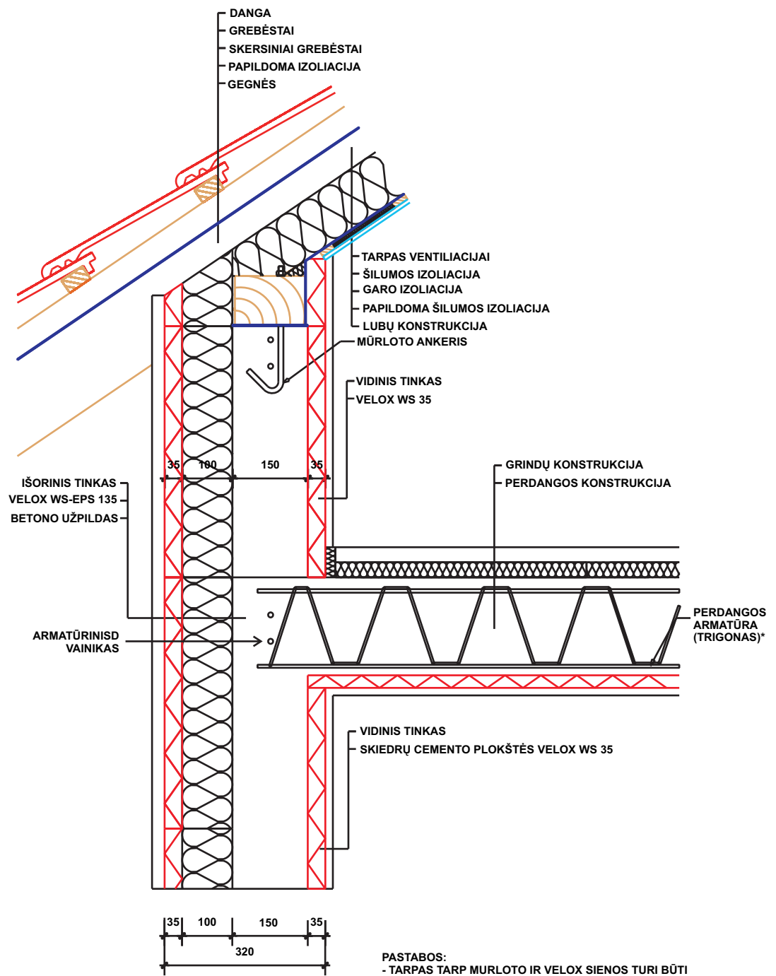
SIENOS STRUKTŪRA VELOX UL 32
