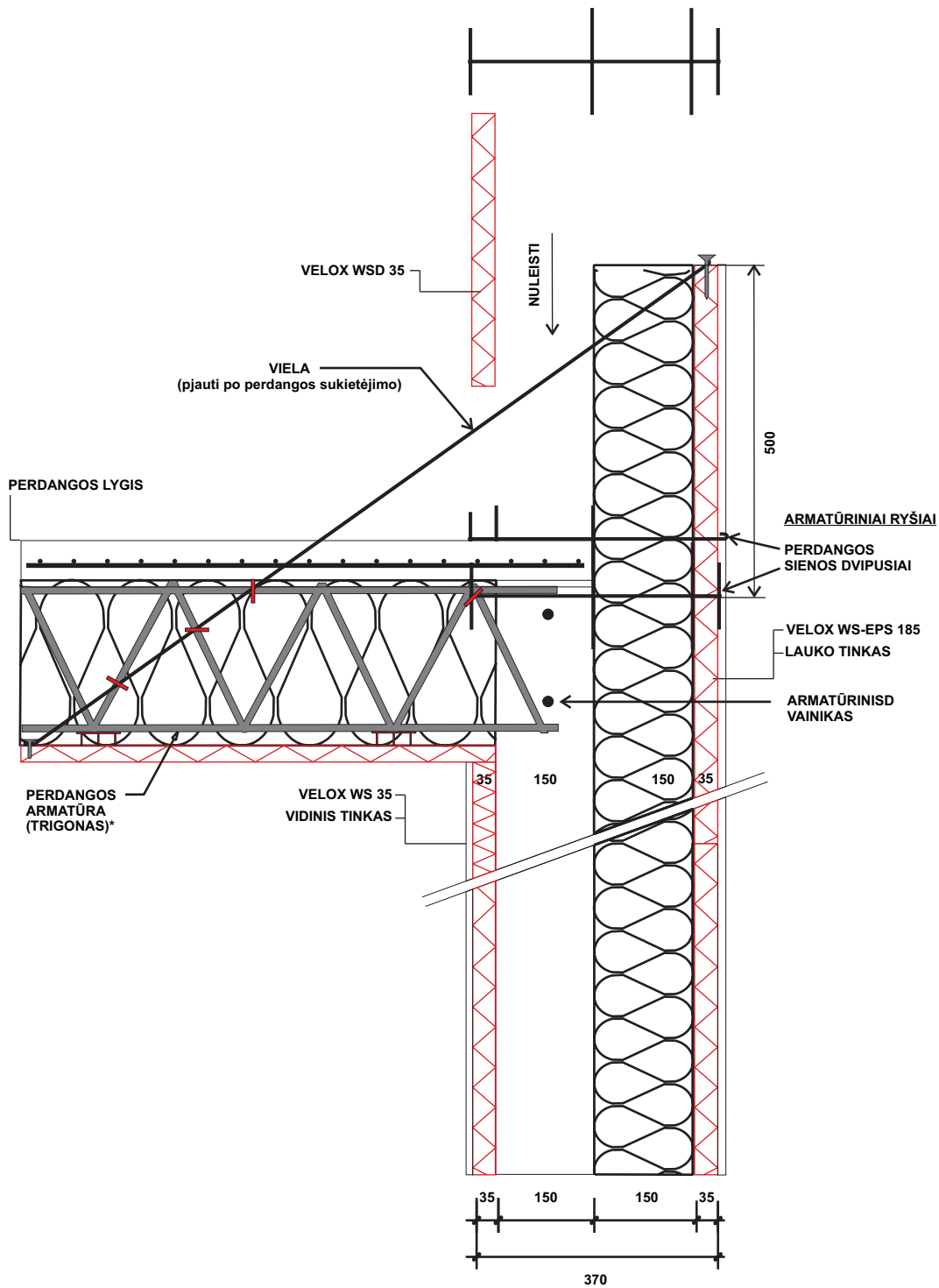
SIENOS STRUKTŪRA VELOX UL 37
