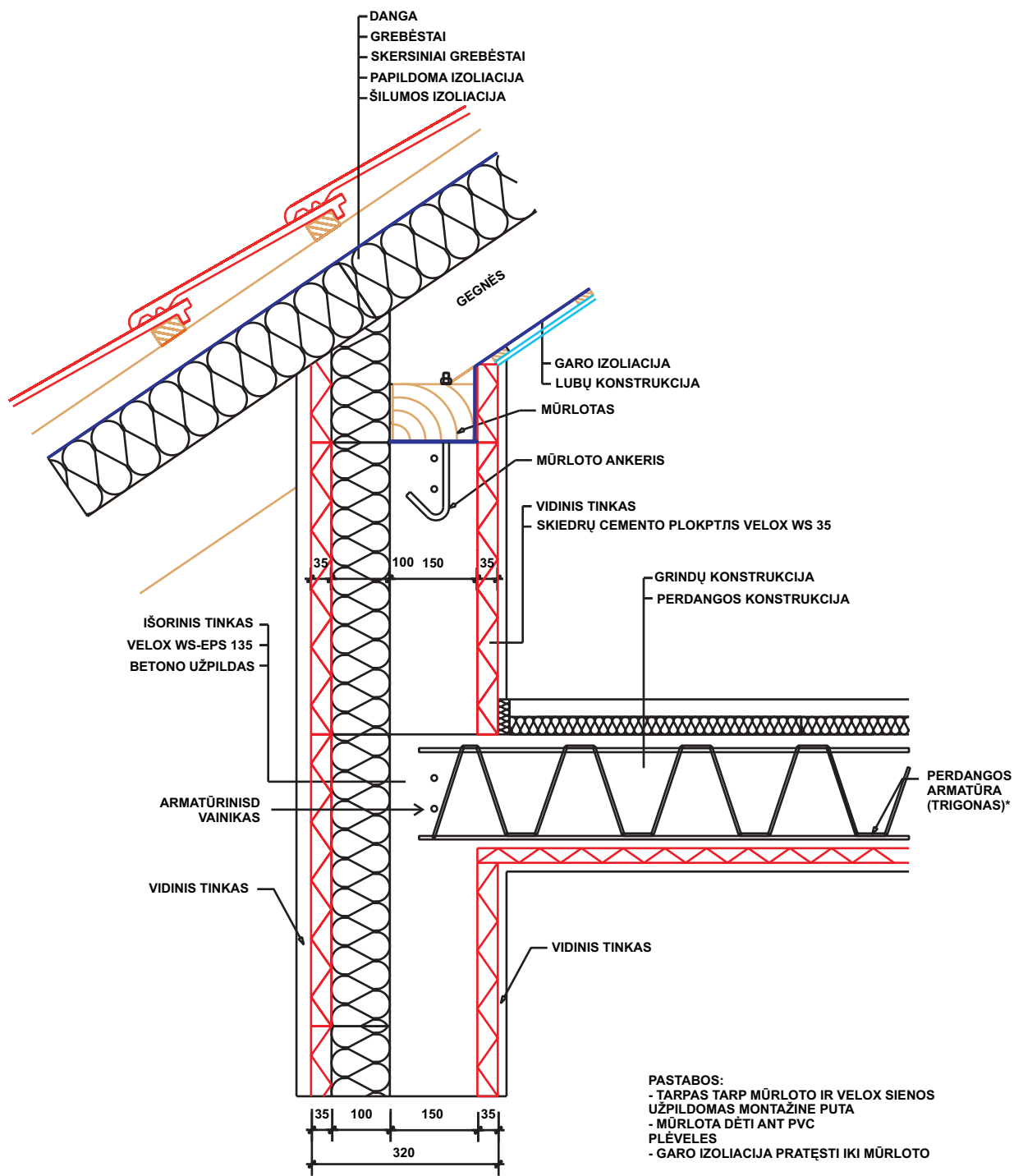
SIENOS STRUKTŪRA VELOX UL32
