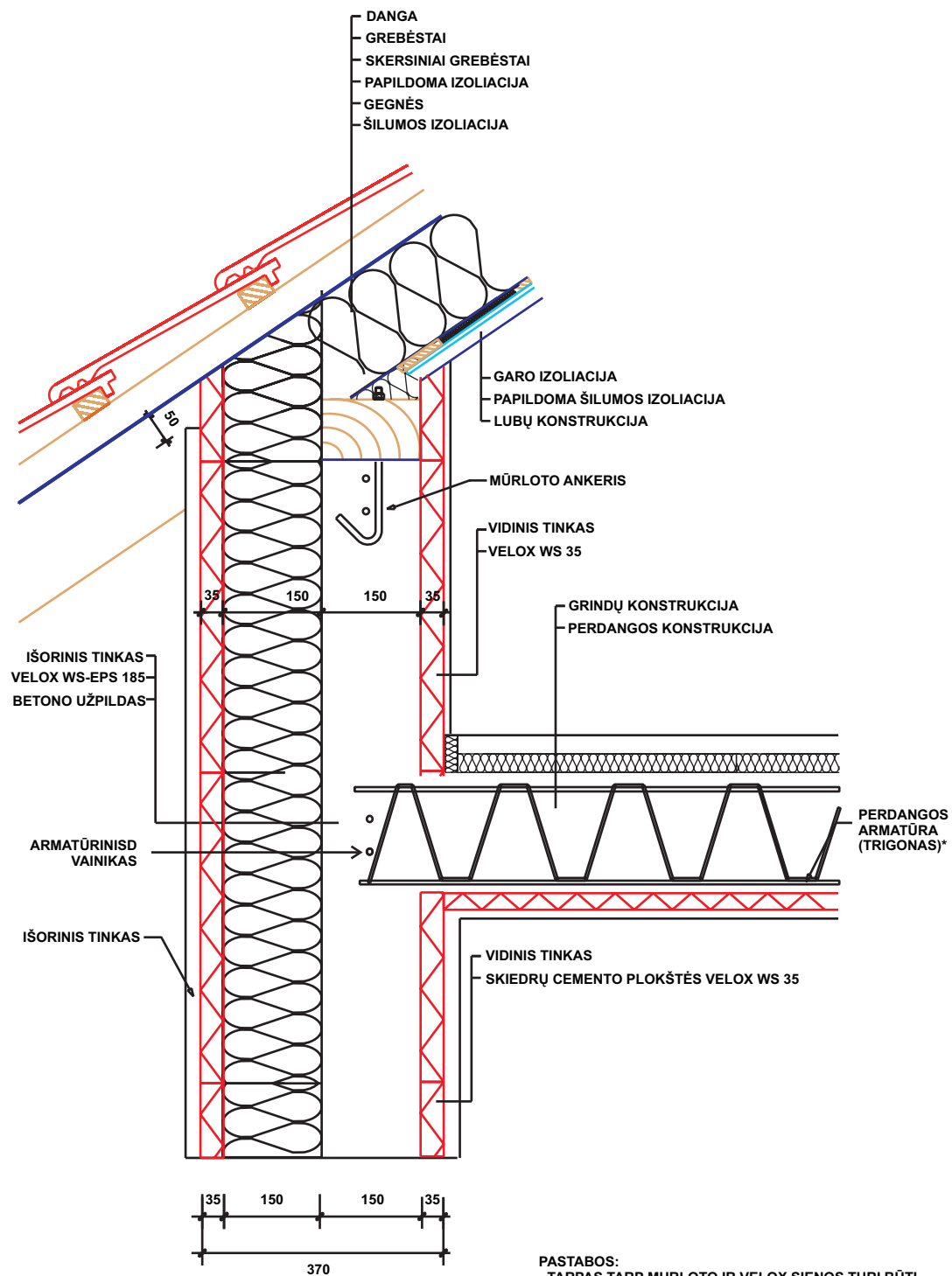
SIENOS STRUKTŪRA VELOX UL 37
