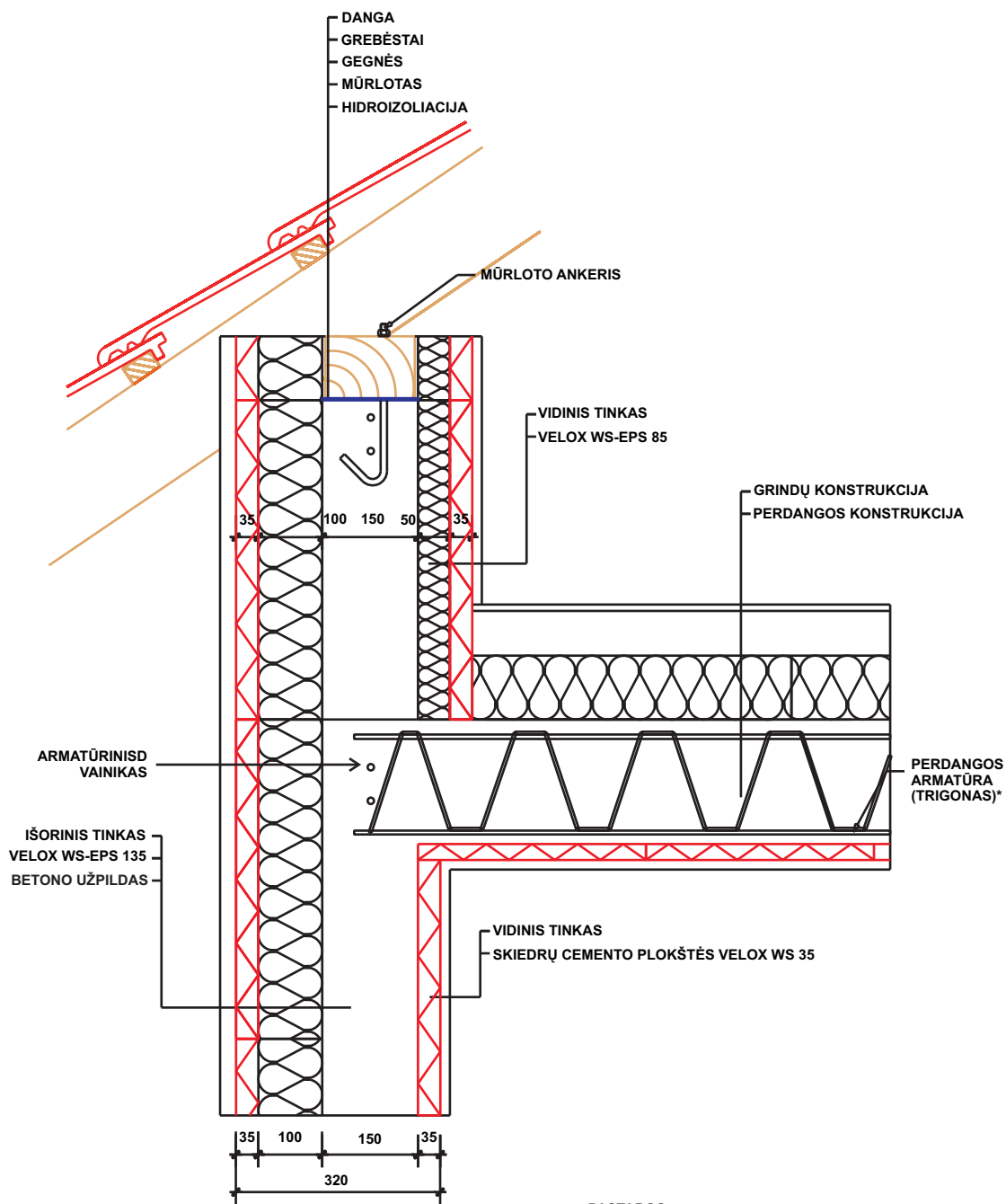
SIENOS STRUKTŪRA VELOX UL 32
