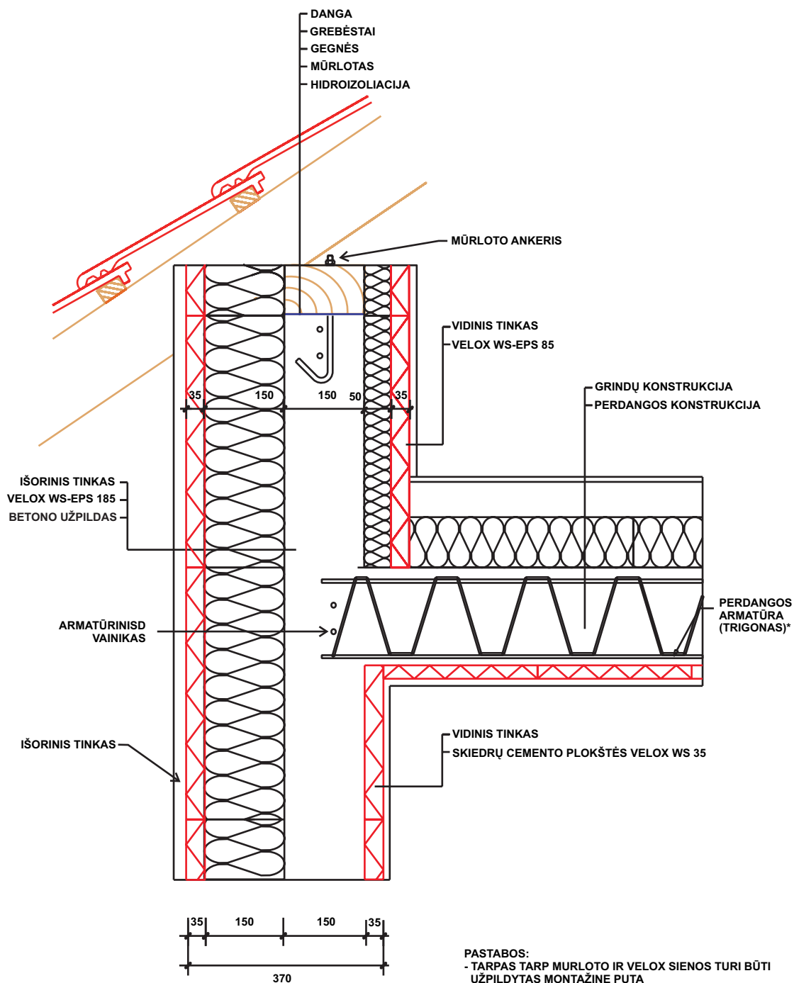
SIENOS STRUKTŪRA VELOX UL 37
