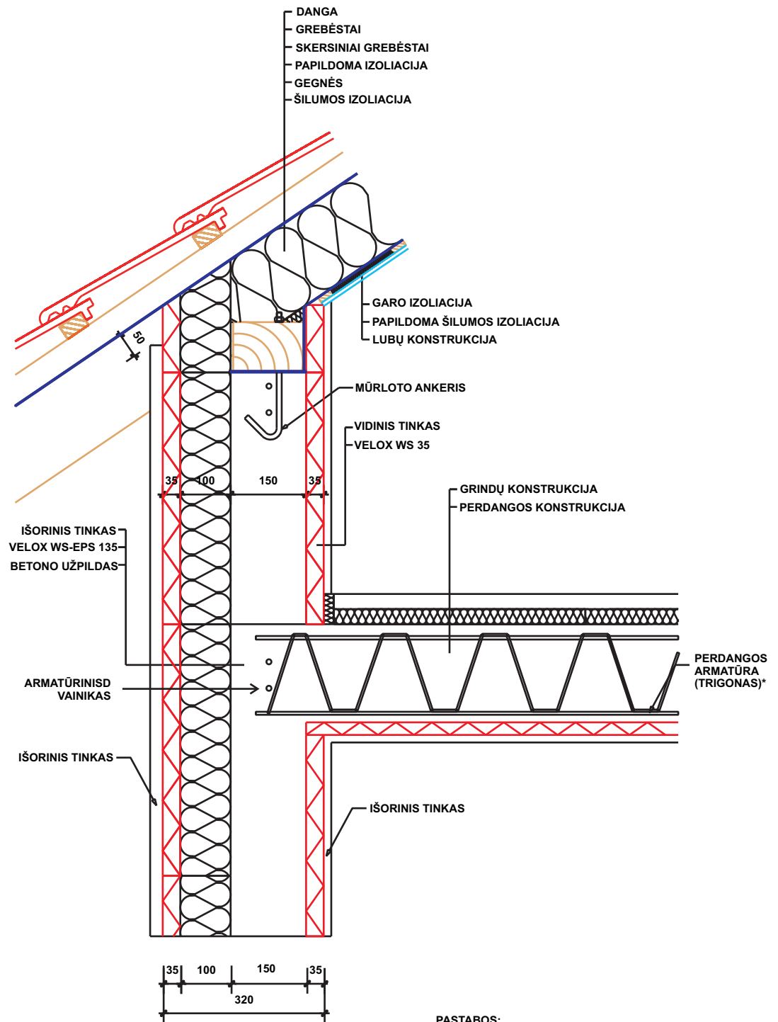
SIENOS STRUKTŪRA VELOX UL 32
