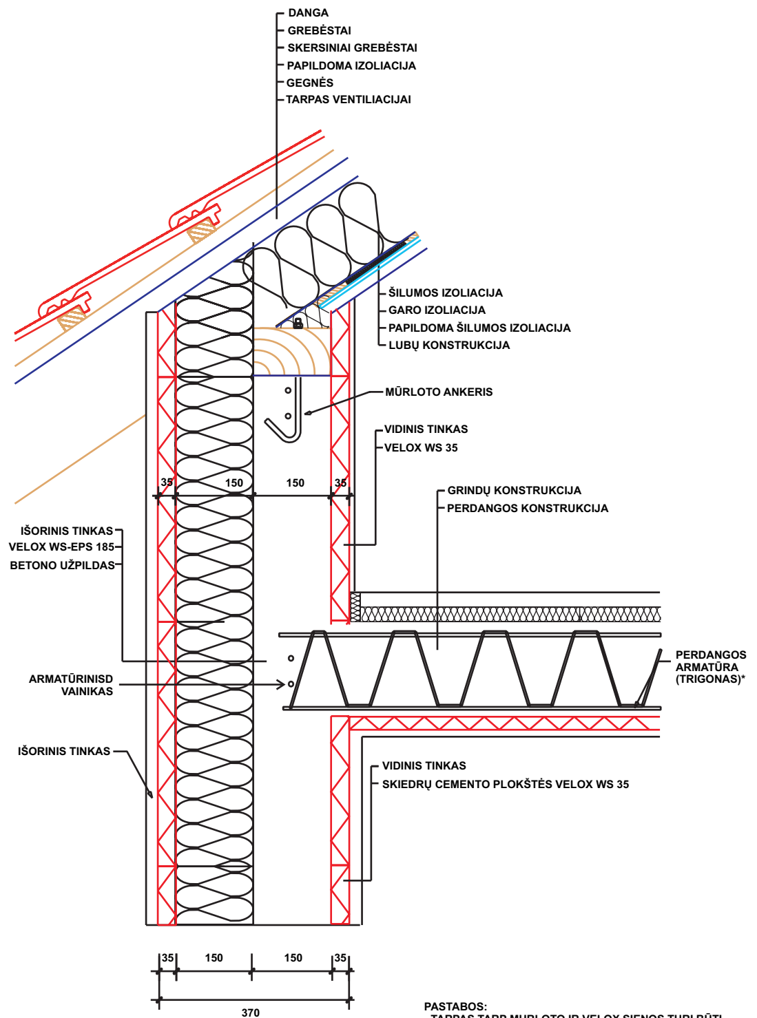
SIENOS STRUKTŪRA VELOX UL 37
