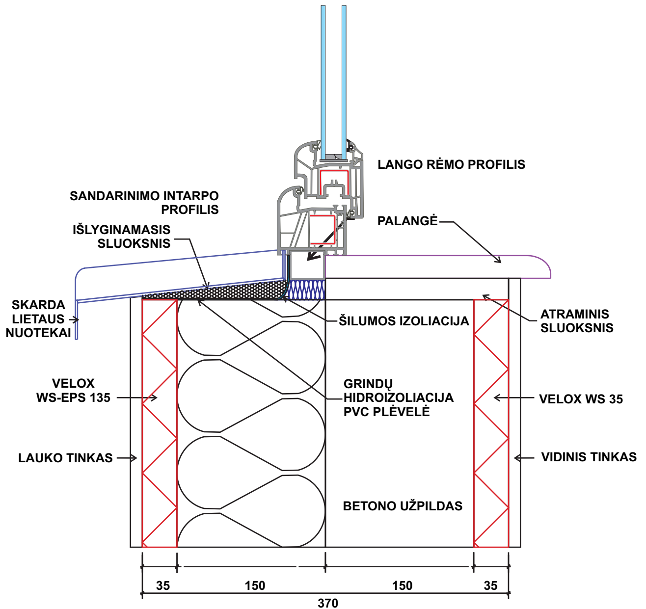
SIENOS STRUKTŪRA VELOX UL 37
