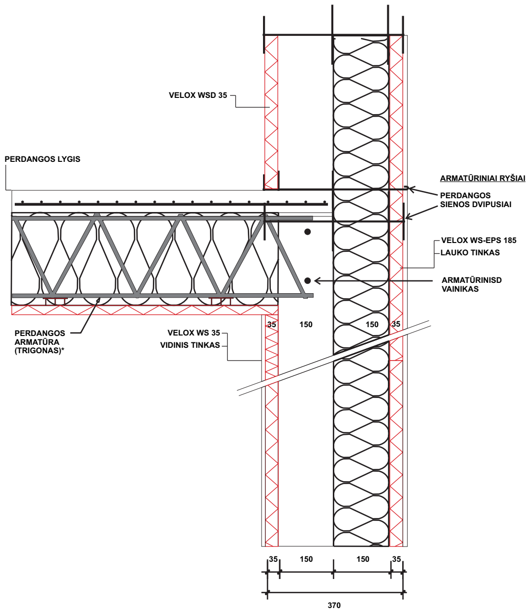
SIENOS STRUKTŪRA VELOX UL 37
