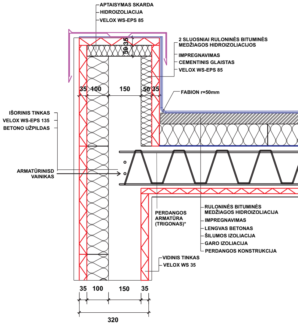
SIENOS STRUKTŪRA VELOX UL 32
