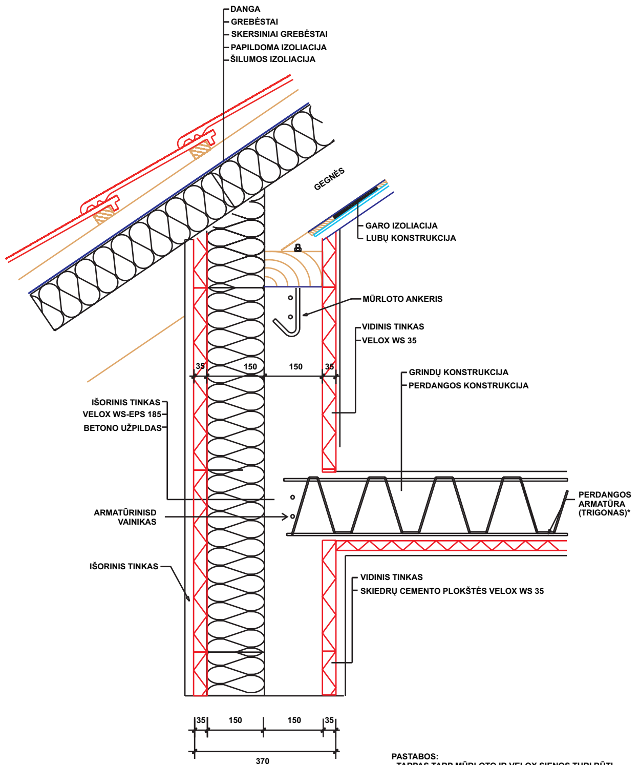
SIENOS STRUKTŪRA VELOX UL 37
